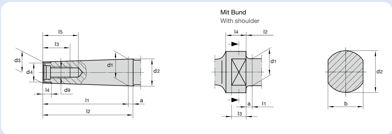
DIN 228 A
