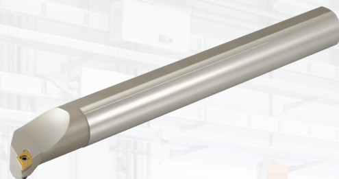
Invändiga svarvhållare för DC. 0702.... skär
